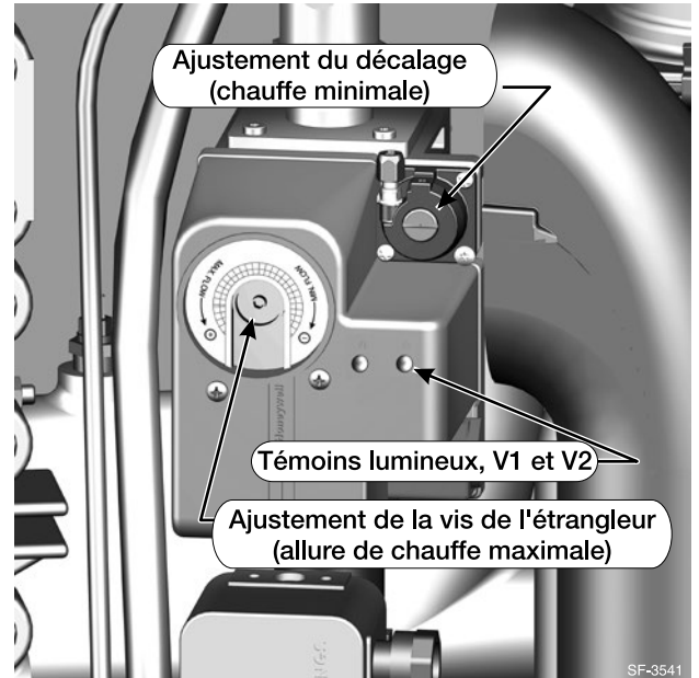
Figure 74 Emplacement de la vis de l'étrangleur (UNIQUEMENT à l'usage d'un technicien qualifié, à l'aide d'appareils de test de combustion étalonnés)
