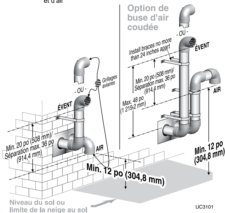
Figure 30 ÉVÈNT DIRECT – Mur latéral – Options de configuration et dégagements minimum par rapport aux terminaisons d'évènt et d'air
