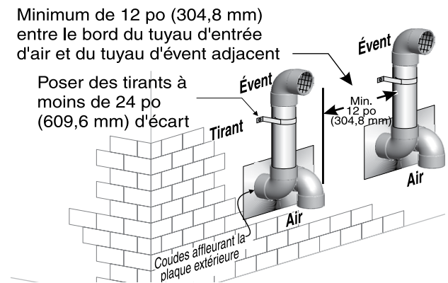
Figure 34 Terminaisons multiples – Tuyaux séparés – Dégagement entre l'événement d'un tuyau et l'entrée d'air du tuyau suivant – Configuration de recharge pour les terminaisons d'air et d'événement
