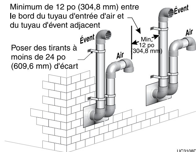
Figure 34 Terminaisons multiples – Tuyaux séparés – Dégagement entre l'événement d'un tuyau et l'entrée d'air du tuyau suivant – Configuration de recharge pour les terminaisons d'air et d'événement
