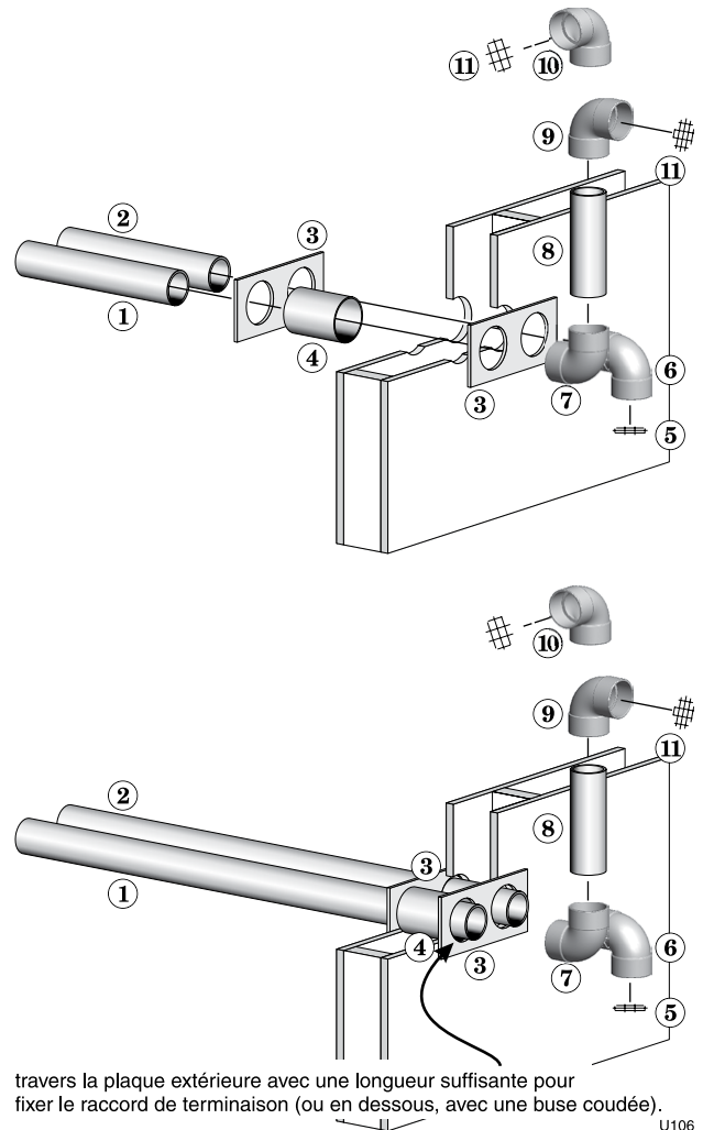
Figure 35 ÉVENT DIRECT – Mur latéral – Ensemble de terminaison (toutes pièces à fournir par l'installateur, sauf les grillages aviaires)
