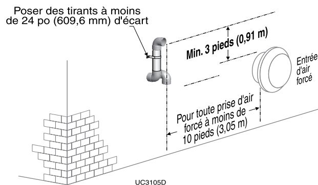
Figure 32 Terminaison sur mur latéral avec tuyaux séparés – Dégagements entre sortie d'évènt et prise d'air forcé
