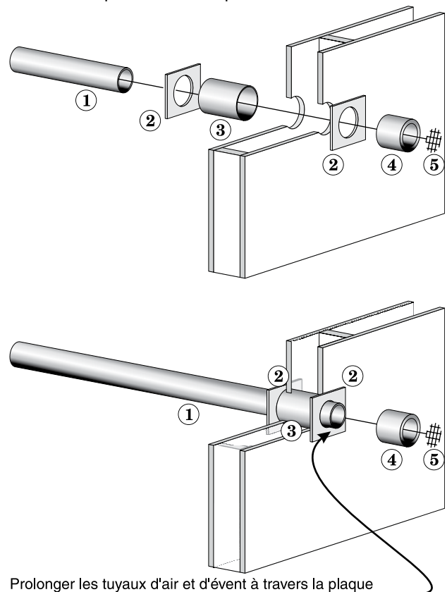
Figure 22 ÉVACUATION DIRECTE – Mur latéral – Ensemble de terminaison – Toutes pièces à fournir par l'installateur
