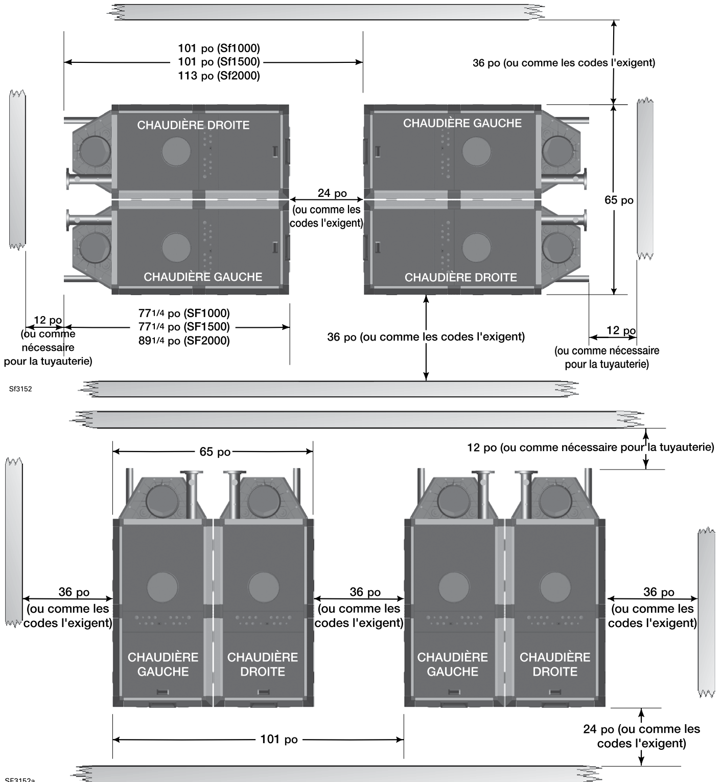
Figure 6 Installation côte à côte de plusieurs chaudières SlimFit (avec l'assemblage de chaudières en configuration à gauche et à droite)
