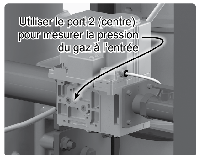
Figure 47 Prise de pression d'admission de la soupape à gaz (disponible des deux côtés de la soupape à gaz).
