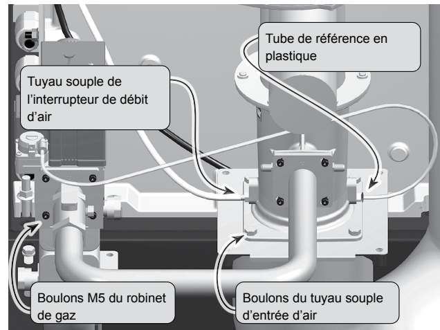
Figure 81 Soupape à gaz et venturi
