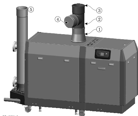
Figure 35 Ventilation directe – Installer un raccord en Té sur l'entrée d'air ou prévoir des moyens de démonter la tuyauterie d'air pour permettre d'accéder au filtre de l'entrée d'air.
