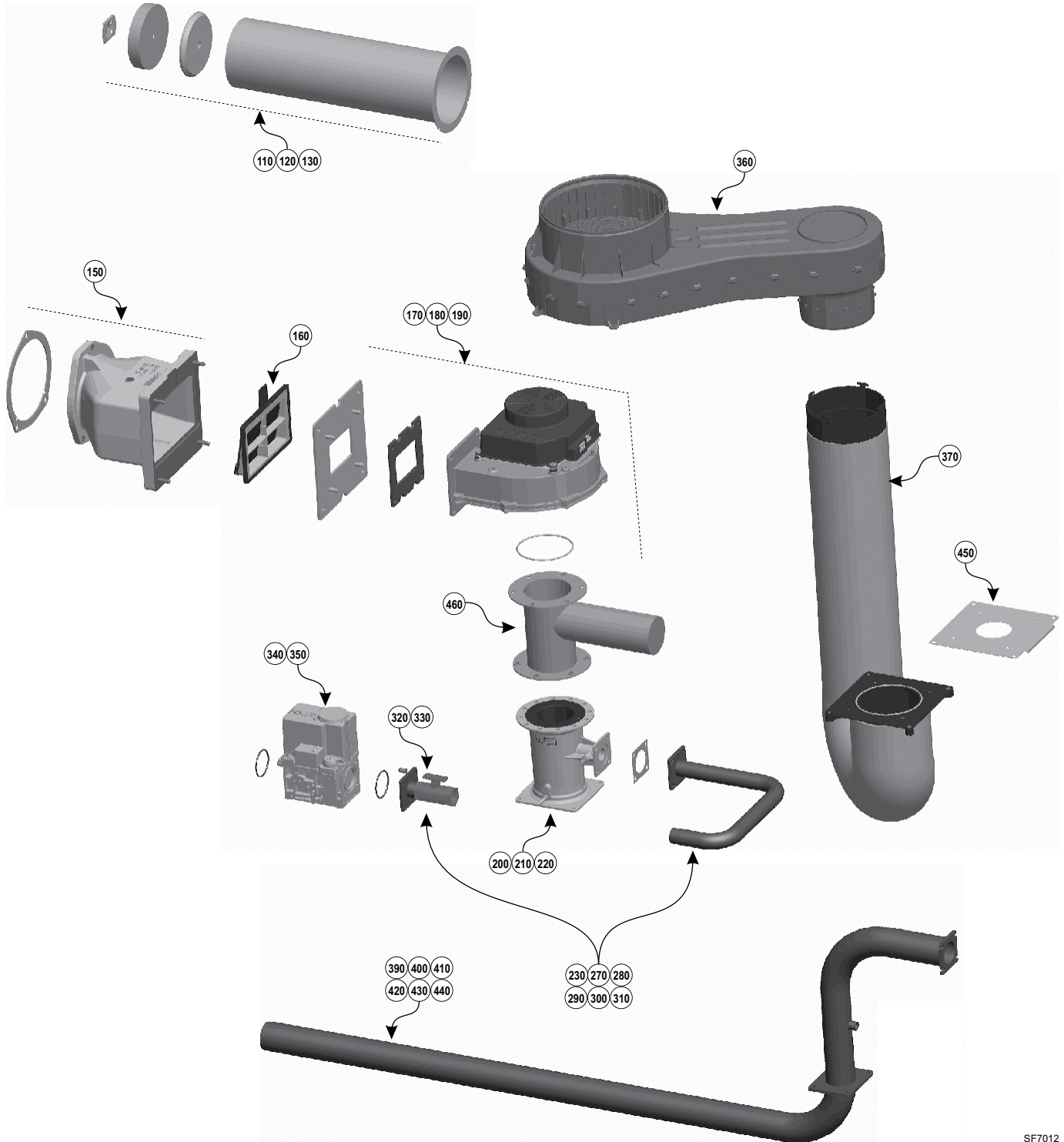
Figure 102 Brûleur, souffleur, venturi et train de gaz
