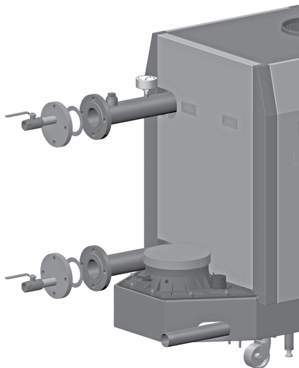
Figure 9 Raccordements des tuyaux pour l'essai hydrostatique – brides, soupapes et joints fournis par l'installateur.
