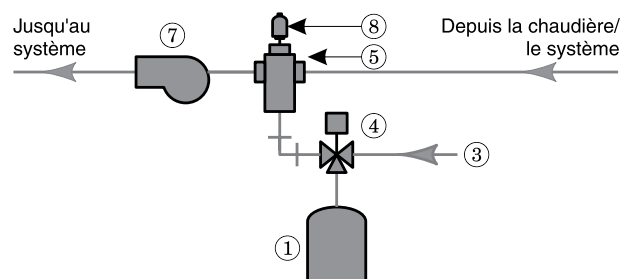
Figure 15 Tuyauterie du réservoir de dilatation – Réservoir de dilatation de type fermé
