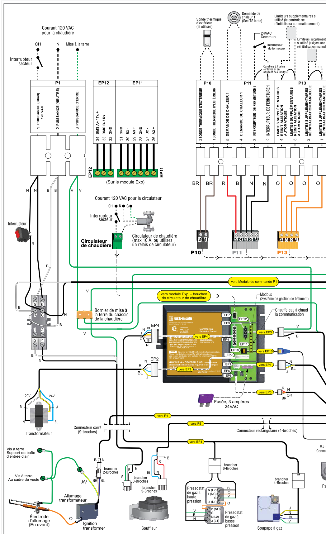
Figure 52 Diagramme de câblage – Chaudières SlimFit (suite à la page suivante)
