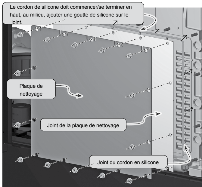
Figure 93 Retirer/réinstaller la plaque de nettoyage.
