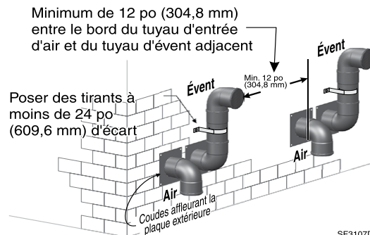
Figure 36 Terminaisons multiples – Dégagement de l'évent d'une à l'entrée d'air de l'autre (dispositions normale et avec coude).
