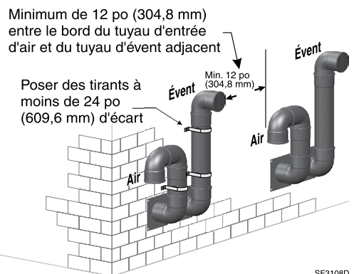
Figure 37 ÉVENT DIRECT – Ensemble de terminaisons dans un mur latéral
