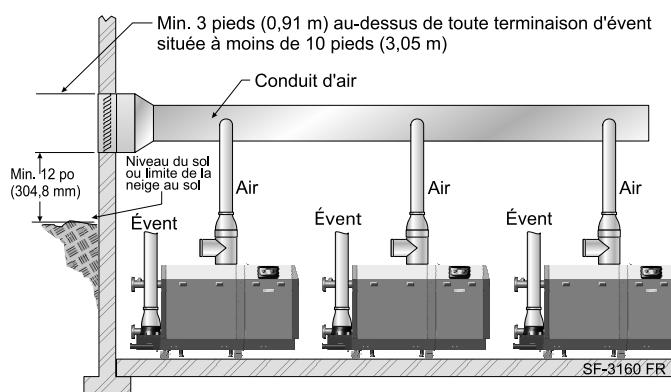
Figure 31 Option d'air comburant relié par collecteur
