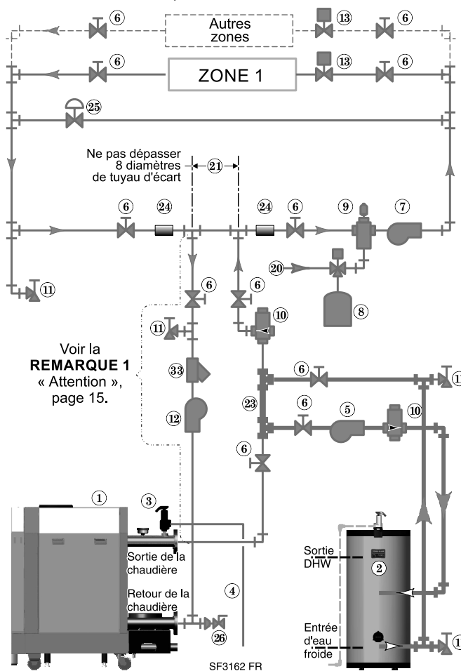
Figure 17 Zonage avec soupapes de secteur plus tuyauterie DHW en option
