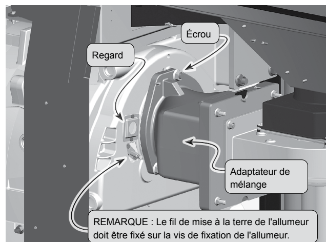
Figure 82 Accès au brûleur
