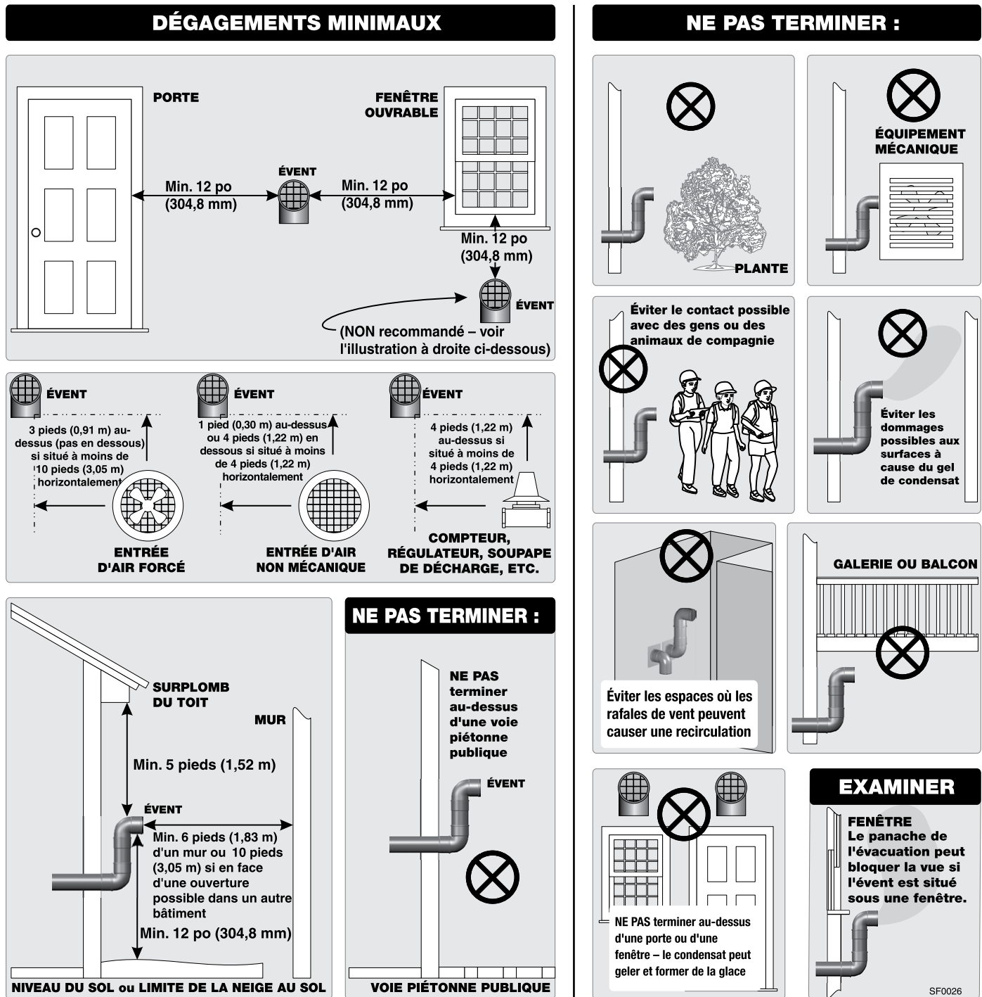
Figure 33 INSTALLATIONS À ÉVENT DIRECT — Exigences pour l'emplacement de terminaison — Dégagements et placement
