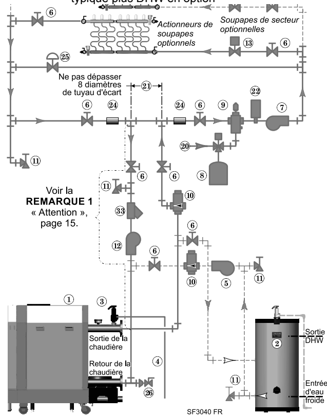
Figure 19 Tuyauterie de système de chauffage radiant typique plus DHW en option
