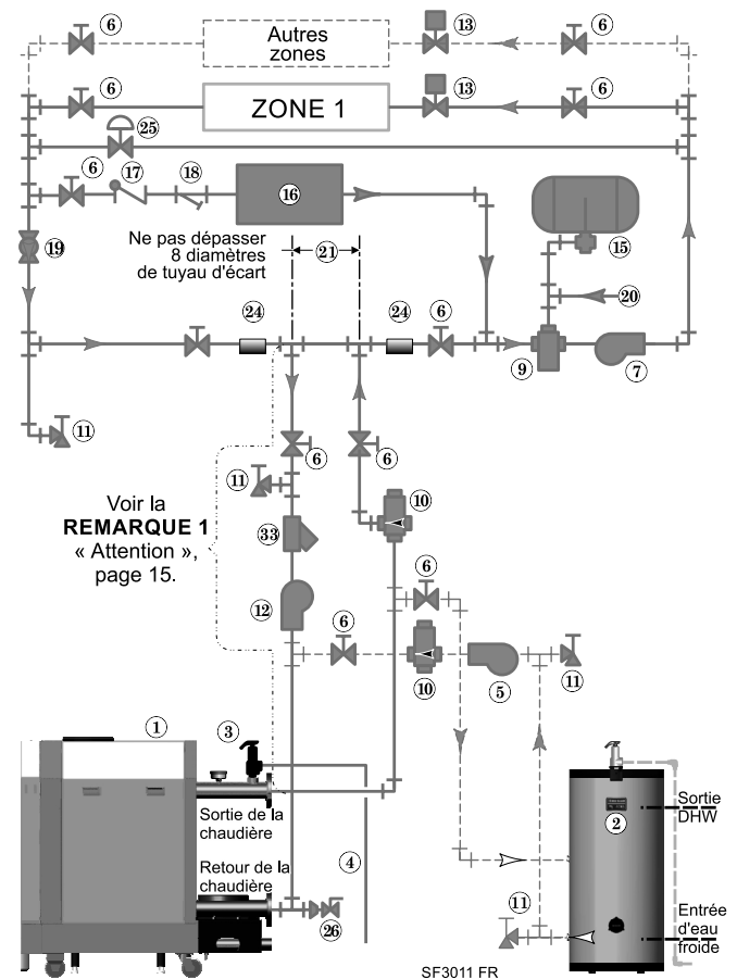
Figure 20 Système à refroidissement d'eau plus tuyauterie DHW en option – tuyauterie primaire/secondaire
