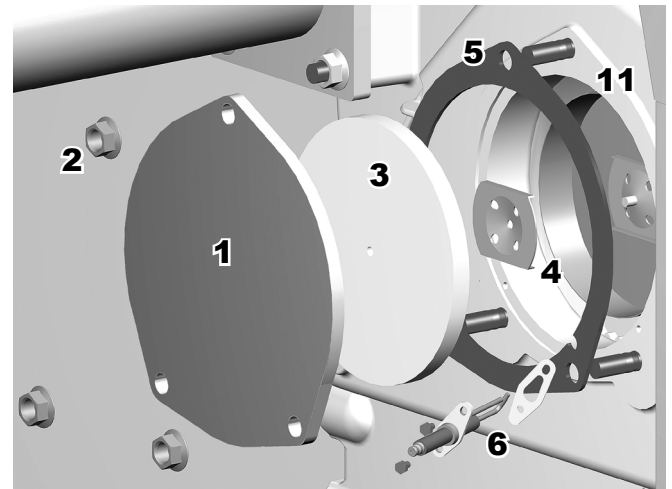
Figure 84 Démontage du couvercle d'accès à la chambre de combustion
