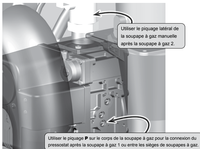
Figure 77 Piquage de pression d'essai de la soupape à gaz
