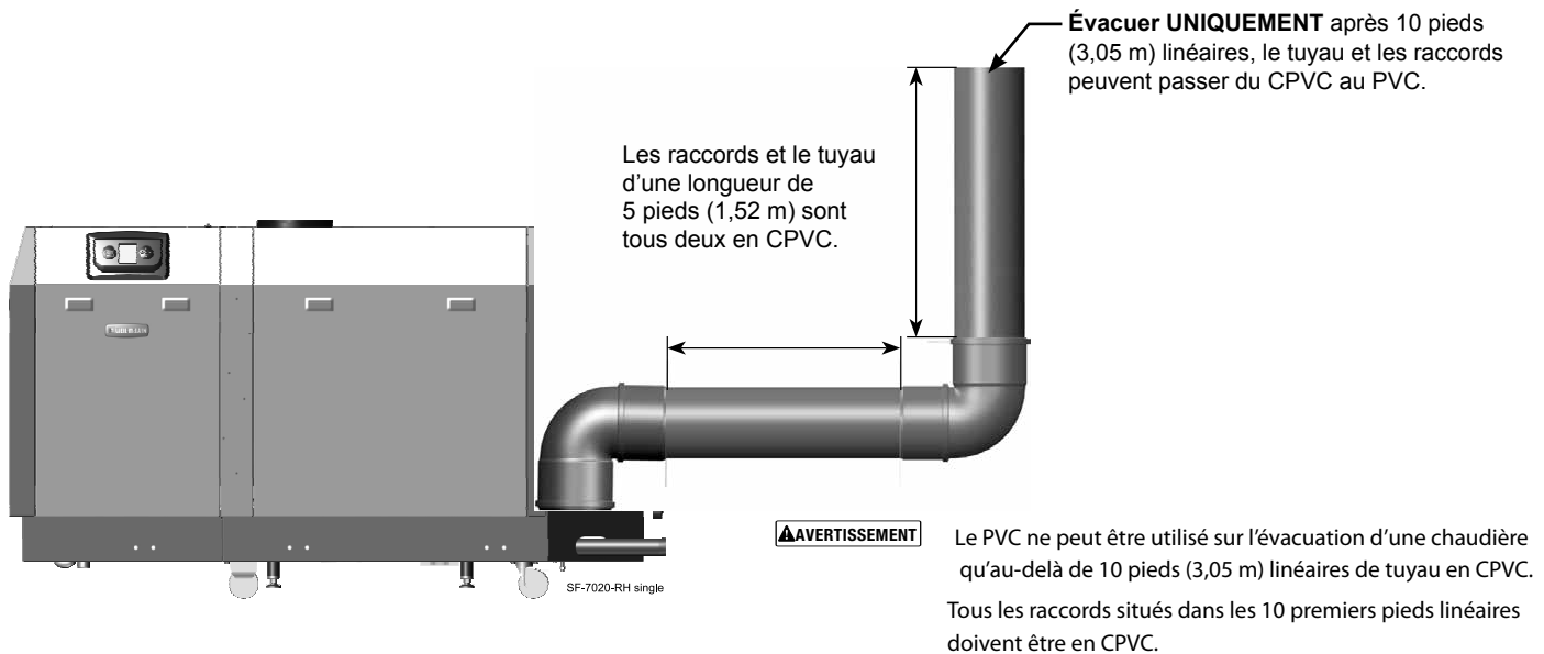
Figure 23 Ventilation en PVC autorisée selon les exigences spécifiées ci-dessous.
