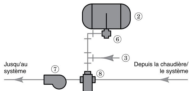
Figure 15 Tuyauterie du réservoir de dilatation – Réservoir de dilatation de type fermé
