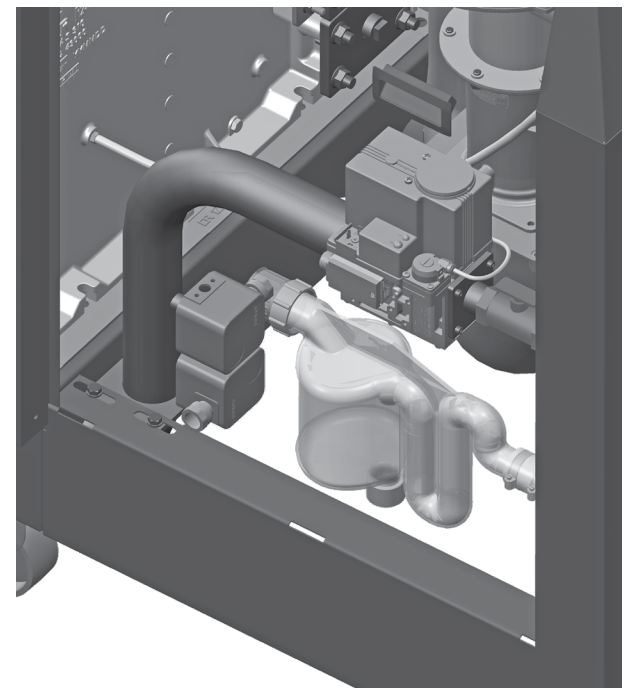
Figure 45 Ensemble du purgeur de condensat, installé
