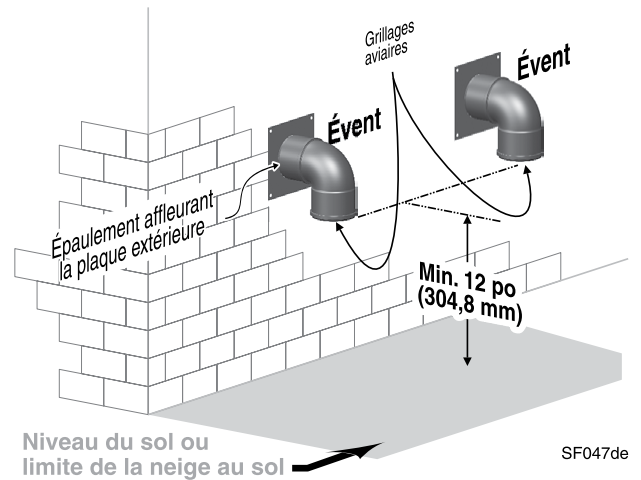
Figure 28 Terminaisons sur mur latéral avec évacuation directe en cas d'installation de plusieurs chaudières (voir la Figure 27, page 33 pour les dégagements requis)
