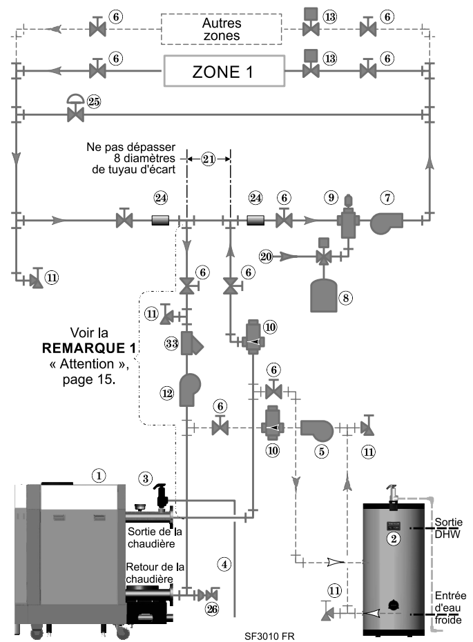
Figure 16 Zonage avec soupapes de secteur plus tuyauterie DHW en option
