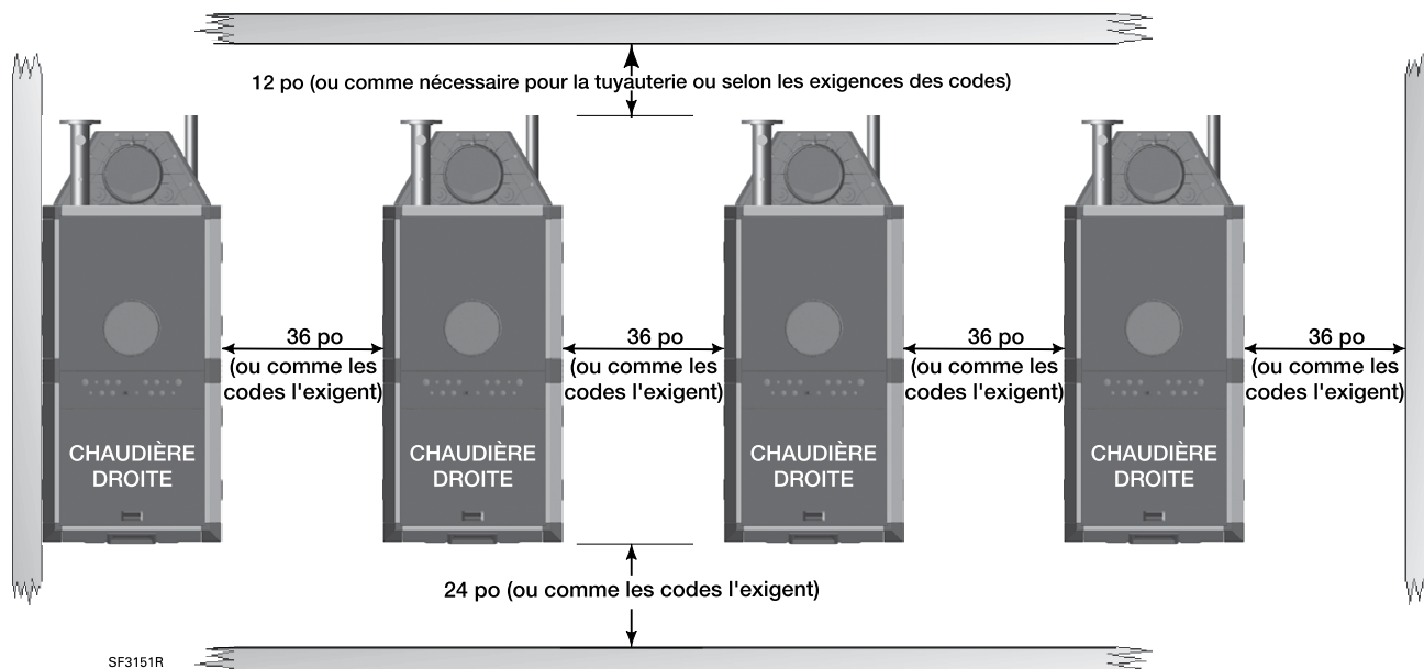
Figure 5 Montage côte à côte de plusieurs chaudières SlimFit – Chaudières en configuration à DROITE seulement
