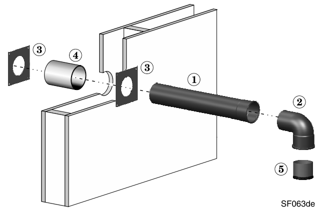
Figure 29 Ensemble de terminaison dans un mur latéral – Installations à évacuation directe
