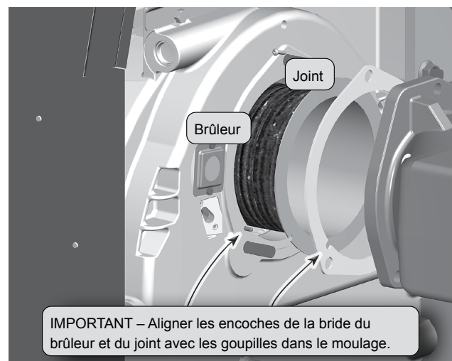
Figure 83 Dépose et remplacement du brûleur
