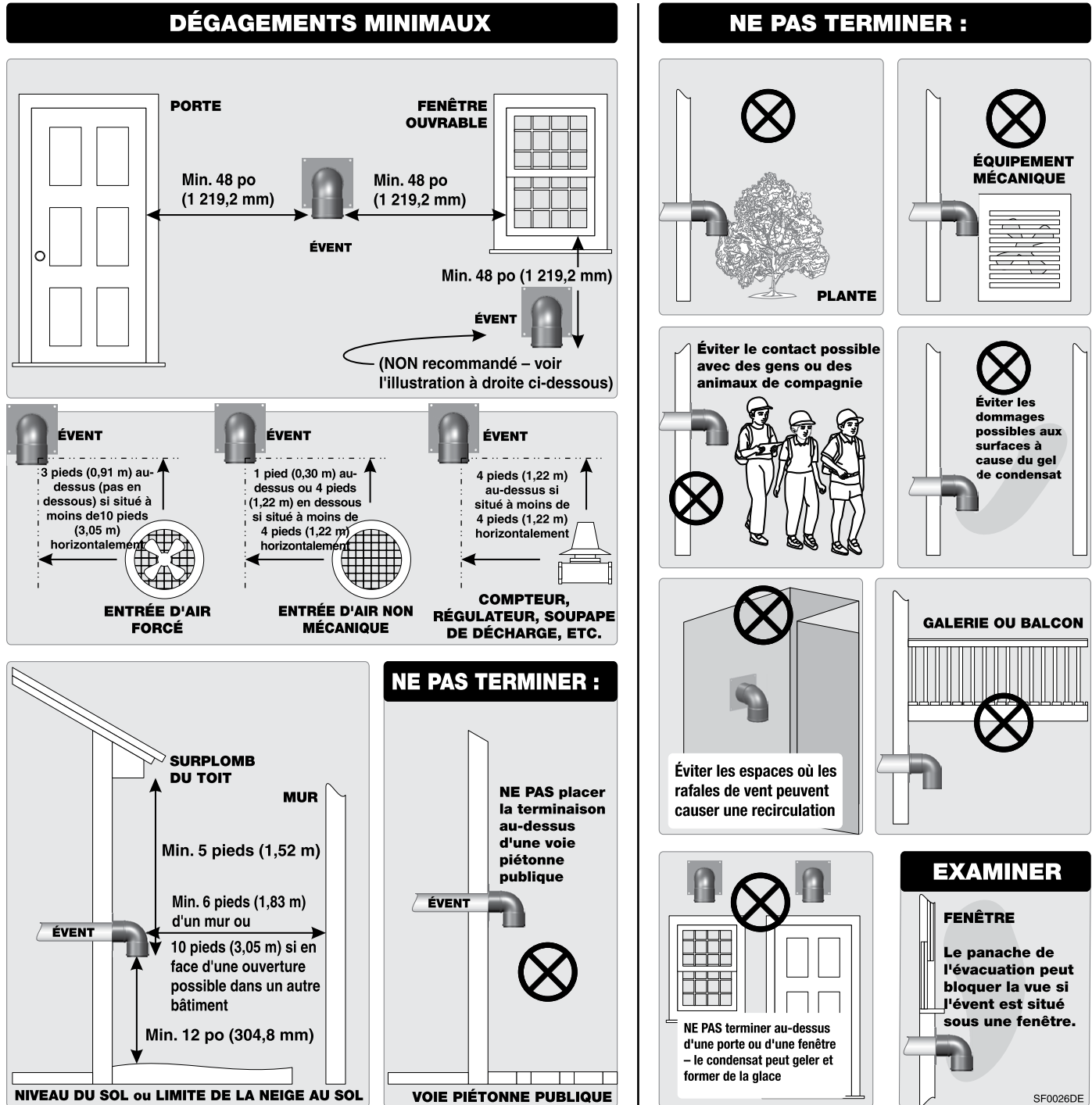
Figure 26 INSTALLATIONS À ÉVACUATION DIRECTE — Exigences pour l'emplacement de terminaison — Dégagements et placement
