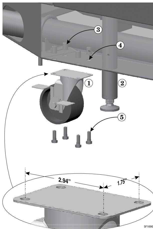
Figure 8 Retrait des roulettes pour permettre le boulonnage de la chaudière aux blocs de montage
