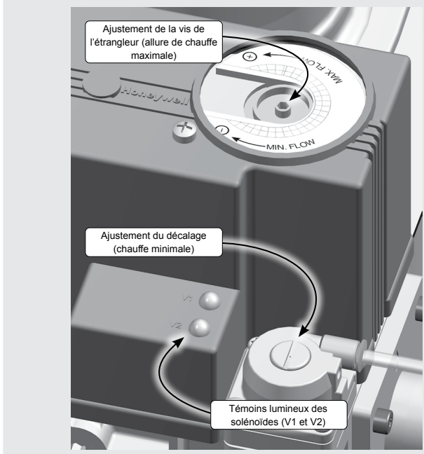
Figure 76 Emplacements d'ajustement de la soupape à gaz ( UNIQUEMENT à l'usage d'un technicien qualifié, à l'aide d'appareils de test de combustion étalonnés )
