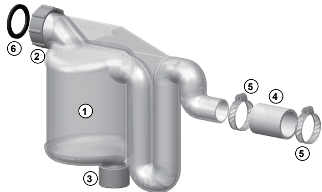
Figure 44 Ensemble du purgeur de condensat
