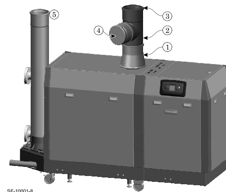
Figure 43 Ventilation directe – Installer un raccord en T sur l'entrée d'air ou prévoir des moyens de démonter la tuyauterie d'air pour permettre d'accéder au filtre de l'entrée d'air.
