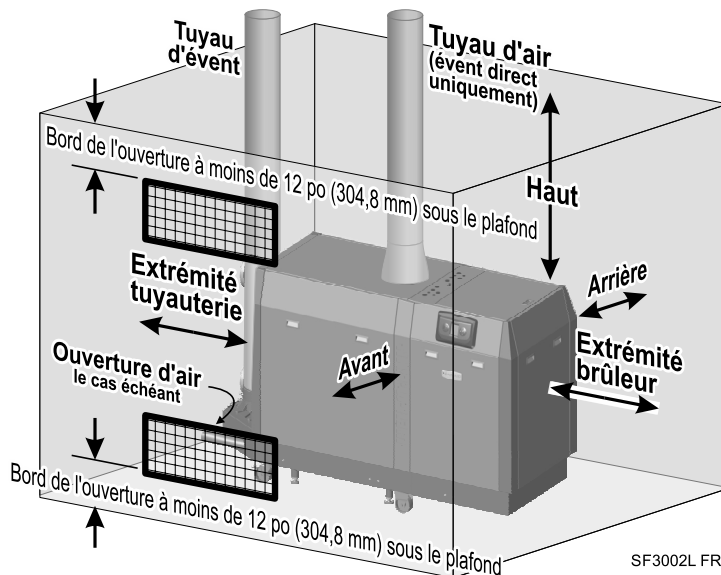
Figure 3 Dégagements pour les chaudières en configuration à DROITE
