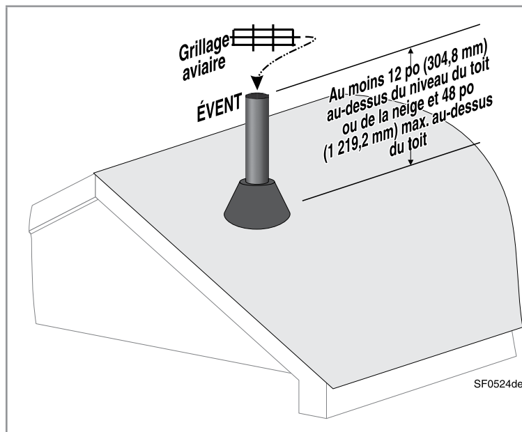
Figure 30 Terminaison verticale de l'évacuation directe
