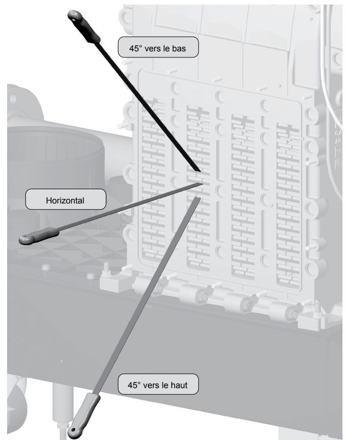
Figure 94 Utilisation de l'outil de nettoyage
