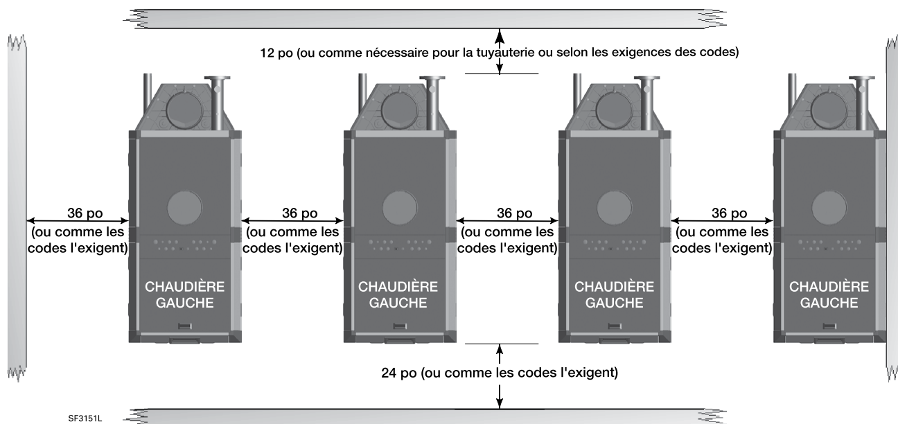
Figure 4 Montage côte à côte de plusieurs chaudières SlimFit – Chaudières en configuration à GAUCHE seulement
