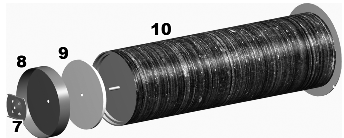
Figure 85 Assemblage de l'extrémité du brûleur
