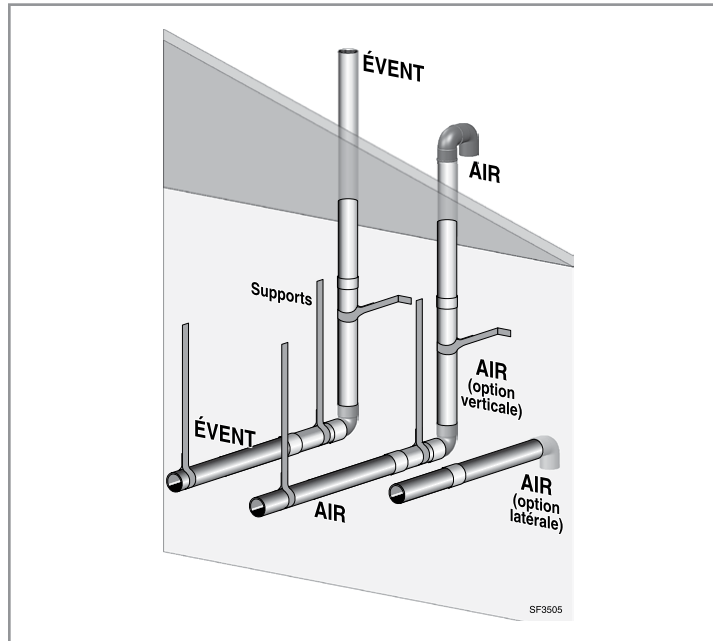
Figure 38 Terminaisons verticales de l'évent direct (la terminaison d'air peut être verticale ou sur un mur latéral, comme illustré ci-dessous).
