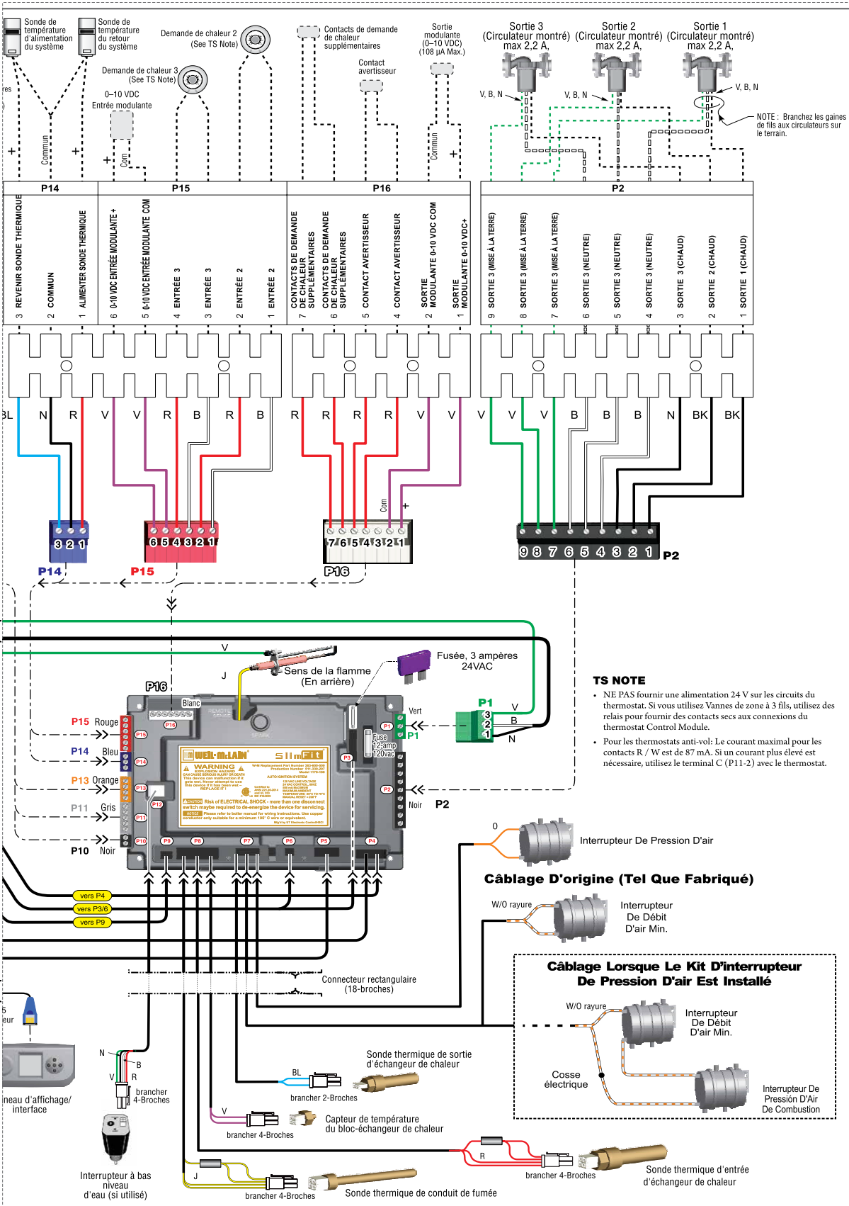
Figure 57 (suite de la page précédente) Diagramme de câblage – Chaudières SlimFit
