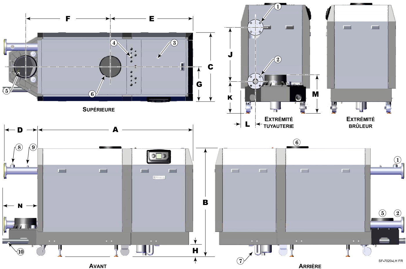
Figure 105 Données dimensionnelles — Configuration d'installation À GAUCHE
