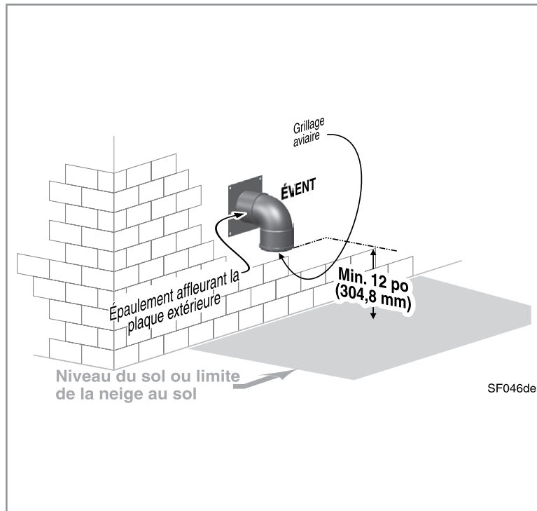
Figure 27 Terminaison d'évacuation directe sur le mur latéral
