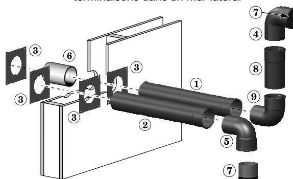
Figure 37 ÉVENT DIRECT – Ensemble de terminaisons dans un mur latéral
