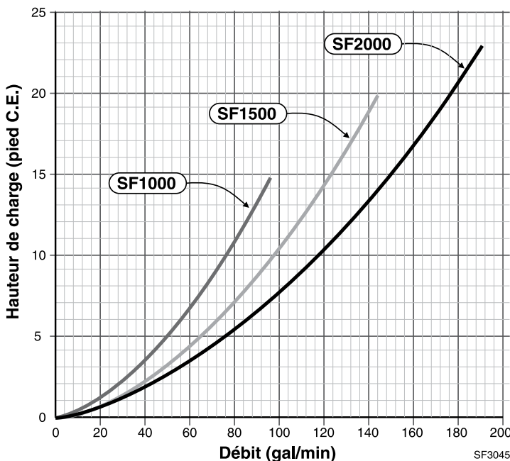
Figure 12 Dimensionnement des tuyaux recommandé vs débit
