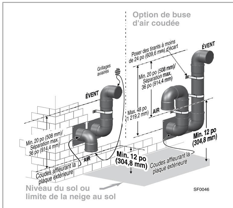
Figure 34 Terminaisons d'évent direct sur le mur latéral – Évén et air
