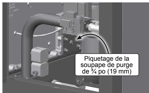
Figure 10 Piquetage de la soupape de purge de la chaudière – emplacement optionnel pour la soupape de purge
