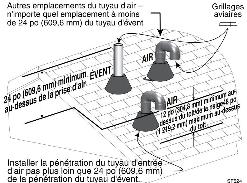
Figure 39 Terminaisons d'air et d'évent verticales.
