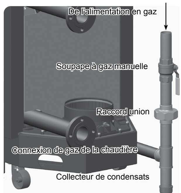
Figure 48 Raccorder la tuyauterie d'alimentation en gaz (tous les raccords et soupapes à gaz sont fournis par l'installateur)
