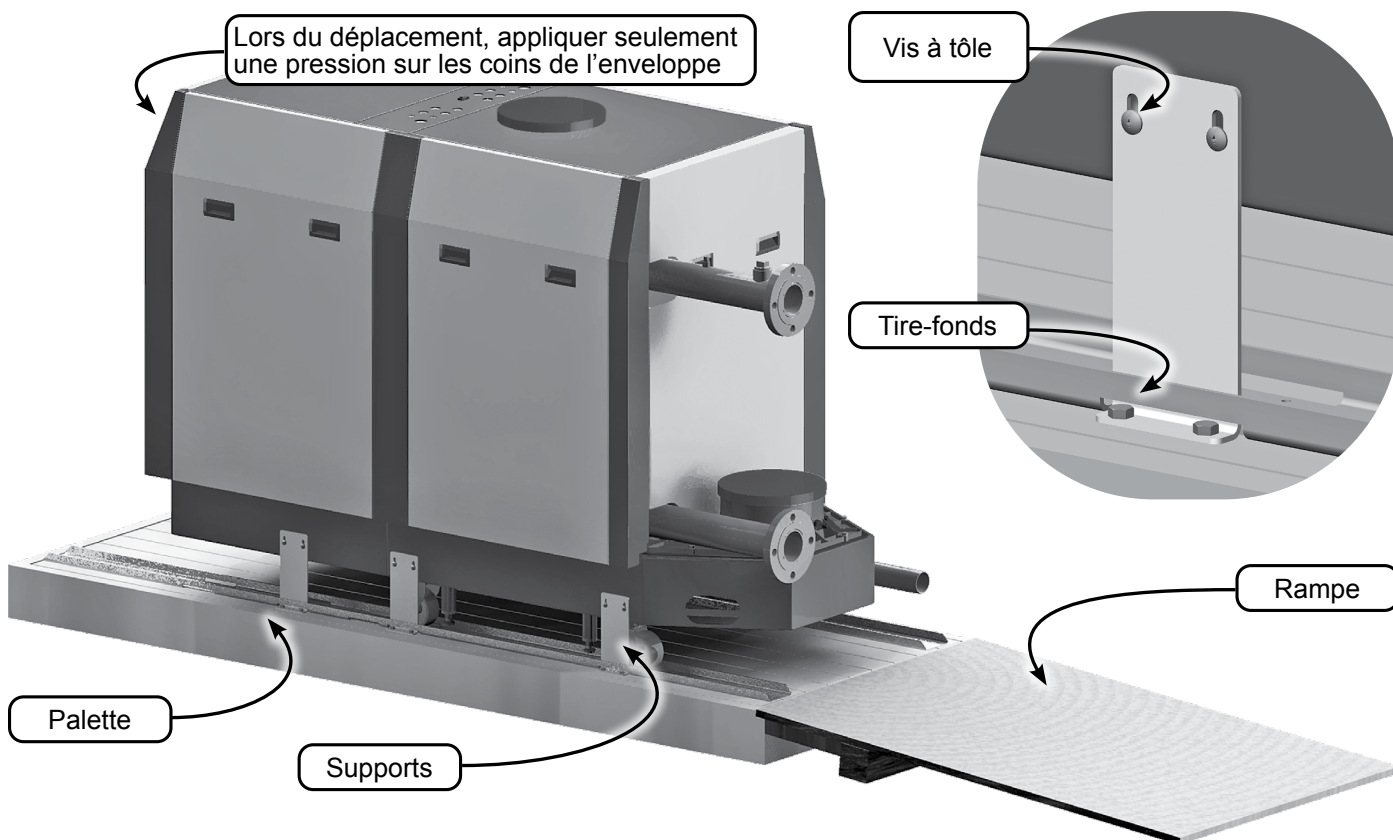
Figure 7 Chaudière SlimFit sur palette, avec rampe en place.
