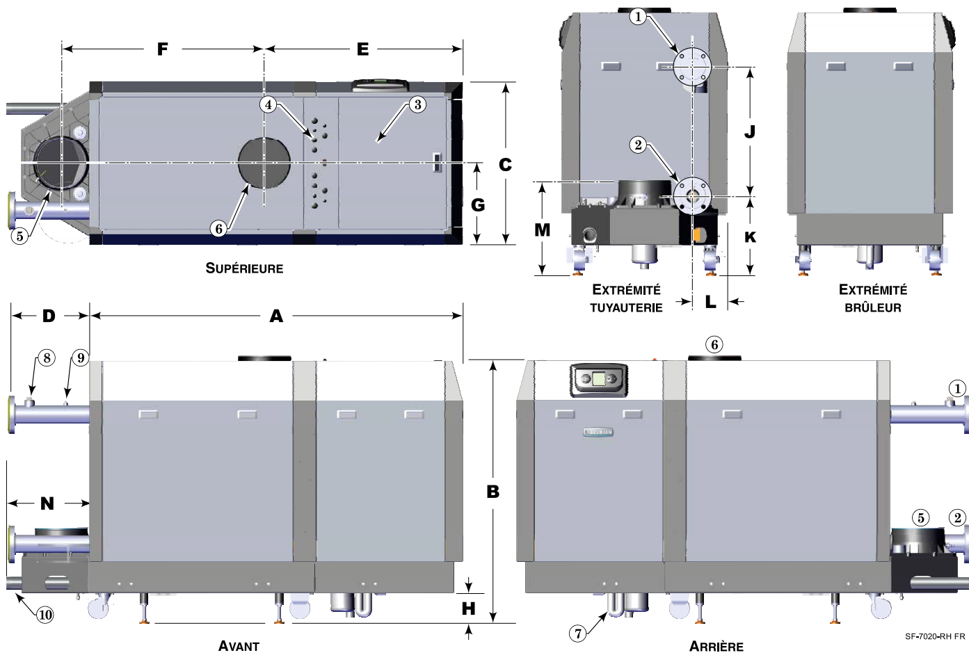
Figure 106 Données dimensionnelles — Configuration d'installation À DROITE
