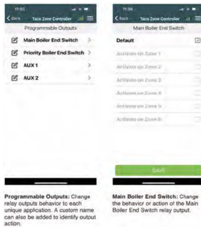
Figure 15 TIU screens
