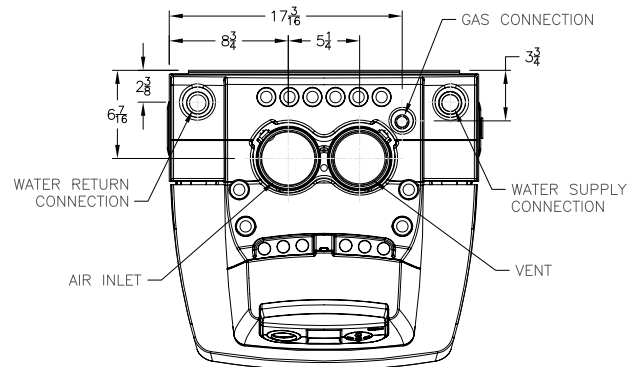
TOP
