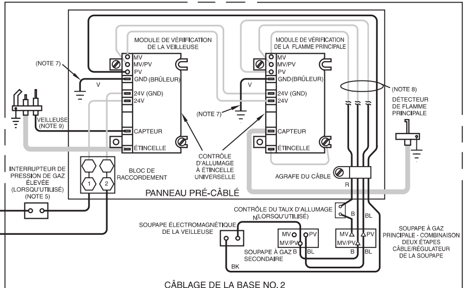
CÂBLAGE DE LA BASE NO. 2 (TAILLES 13 À 23)
