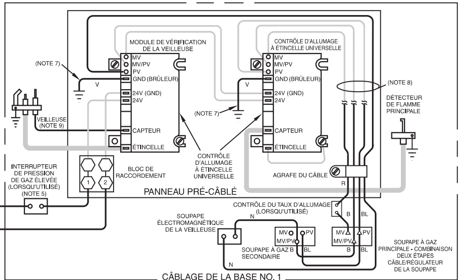
CÂBLAGE DE LA BASE NO. 1 (TAILLES 6 À 23)
