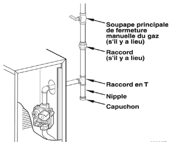
Illustration 14 Tuyauterie d'alimentation en gaz
