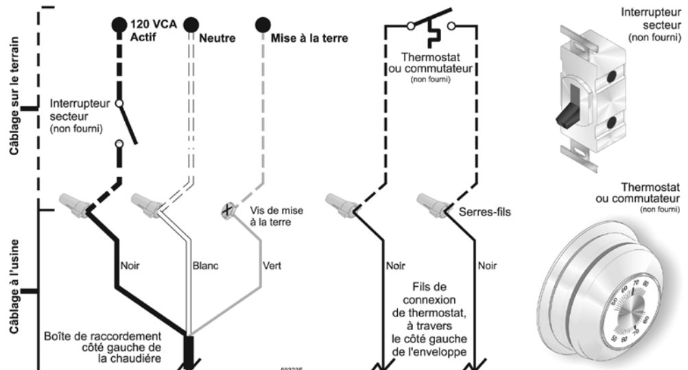
Illustration 15 Connexions de câblage sur le terrain — Interrupteur de secteur et thermostat (ou commutateur) fourni par l'installateur
