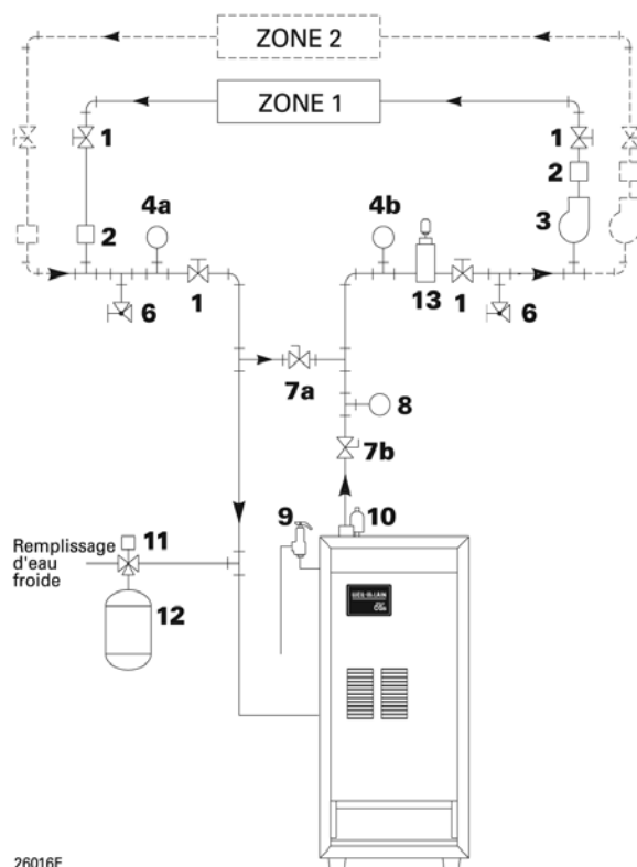
Illustration 10 Tuyauterie de dérivation de chaudière Zonage avec circulateurs (Alternative à la tuyauterie primaire/secondaire Illustrations 8 et 9)
