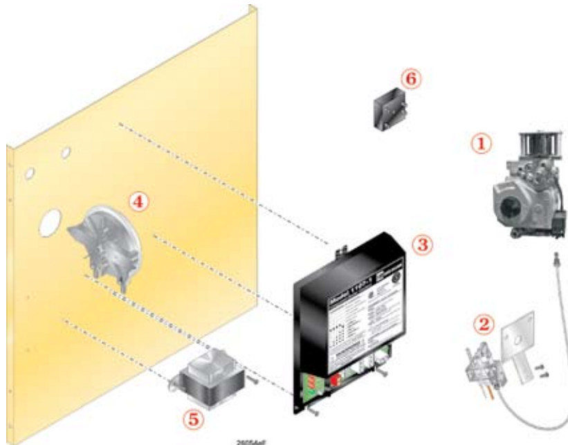
Illustration 30 Pièces de contrôle du gaz
