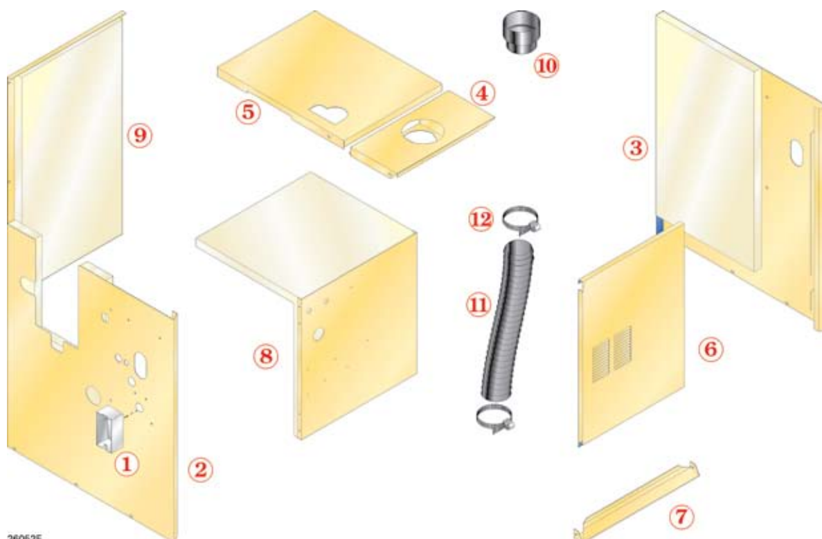
Illustration 28 Pièces de l'enveloppe
