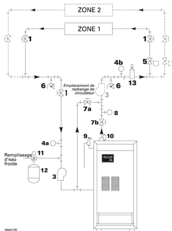
Illustration 11 Tuyauterie de dérivation de chaudière Zonage avec soupapes de zone (Alternative à la tuyauterie primaire/secondaire Illustrations 8 et 9)
