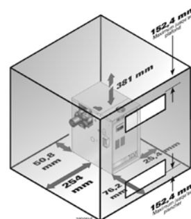
Illustration 2 Dégagements minimum pour les endroits à l'étroit
