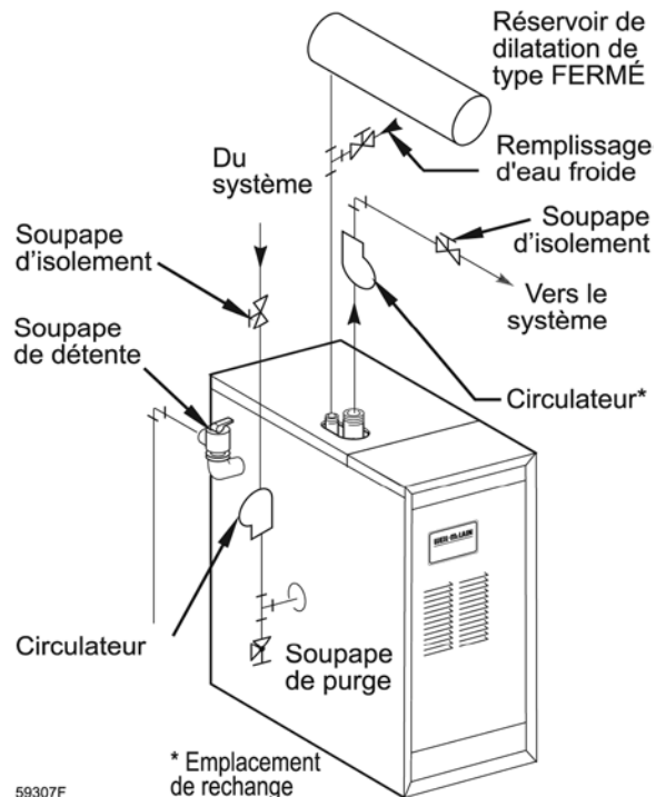
Illustration 5 Réservoir de dilatation de type fermé Tuyauterie vers un système à une seule zone Voir le tableau 3 pour les dimensions de tuyauterie.
