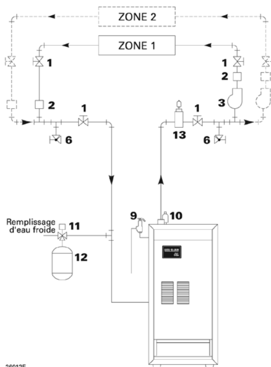
Illustration 6 Zonage avec circulateurs — eau de retour à 54,4 °C ou plus.
