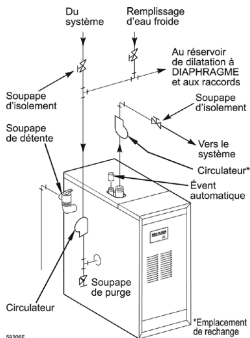
Illustration 4 Réservoir de dilatation de type diaphragme ou vessie Tuyauterie vers un système à une seule zone Voir le tableau 3 pour les dimensions de tuyauterie.
