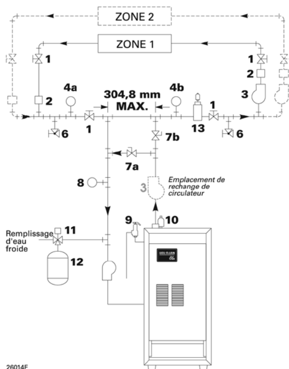
Illustration 8 Tuyauterie primaire/secondaire Zonage avec circulateurs
