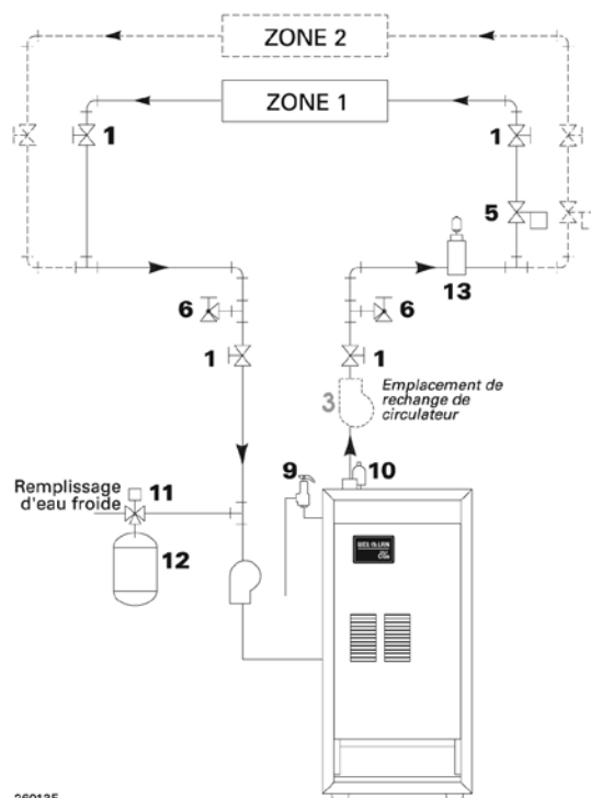
Illustration 7 Zonage avec soupapes de zone — eau de retour à 54,4 °C ou plus.
