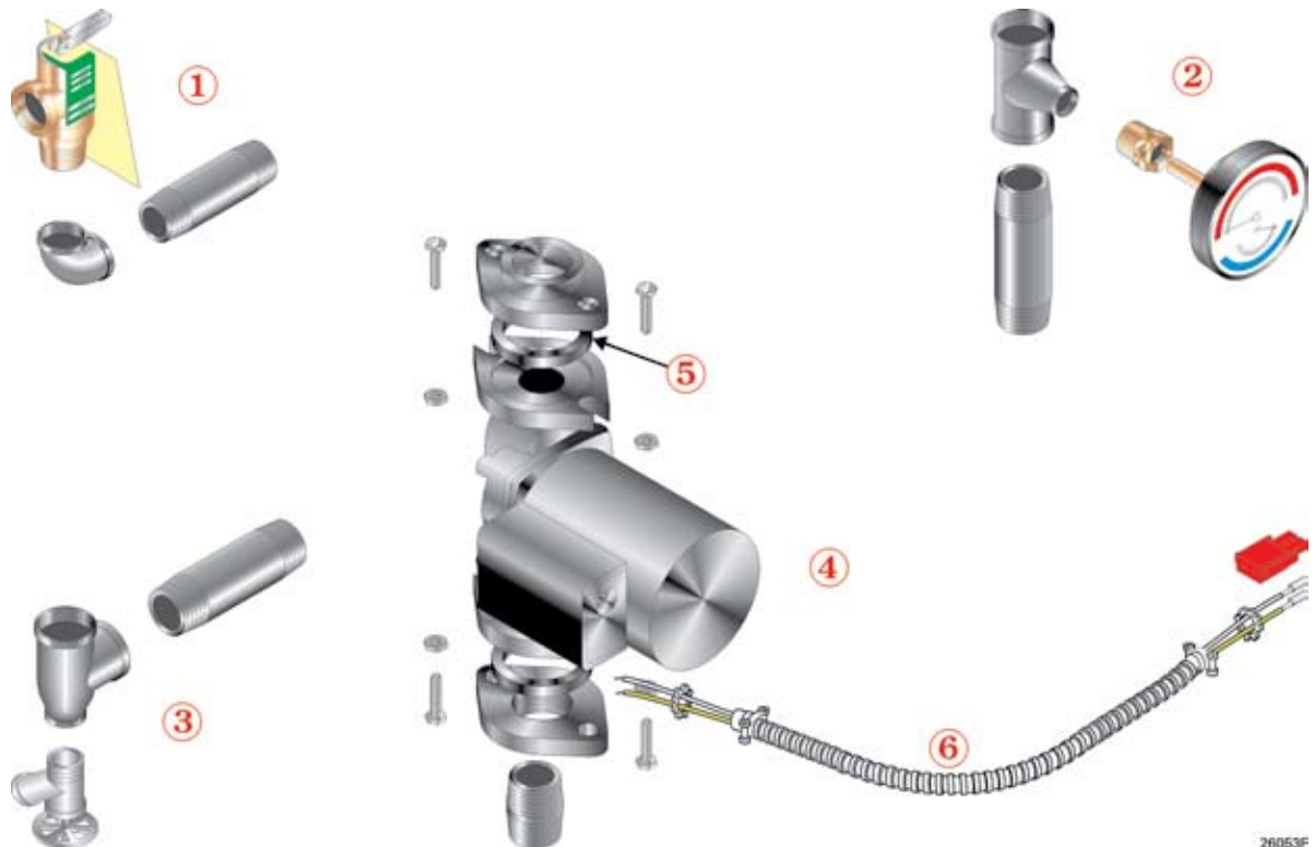
Illustration 29 Pièces d'éléments internes
