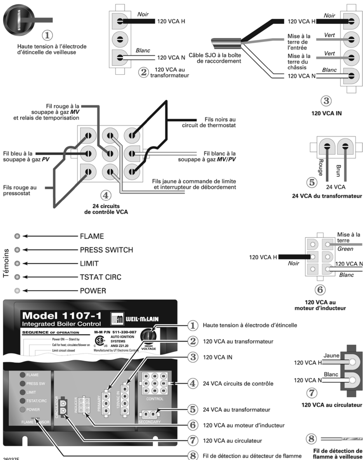
Illustration 25 Connexions de module de contrôle
