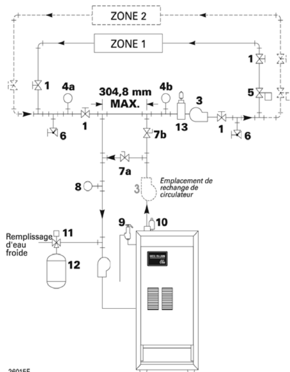
Illustration 9 Tuyauterie primaire/secondaire Zonage avec soupapes de zone
