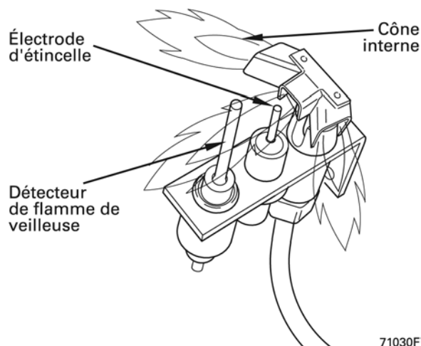
Illustration 16 Flamme typique d'un brûleur de veilleuse
