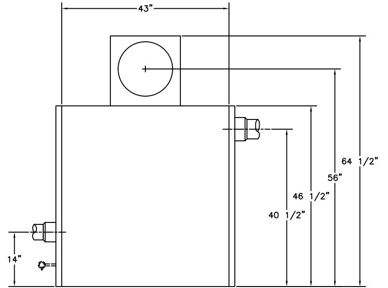
TOP
