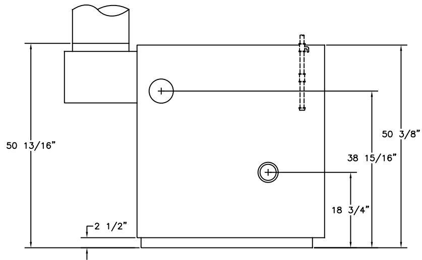
LEFT
