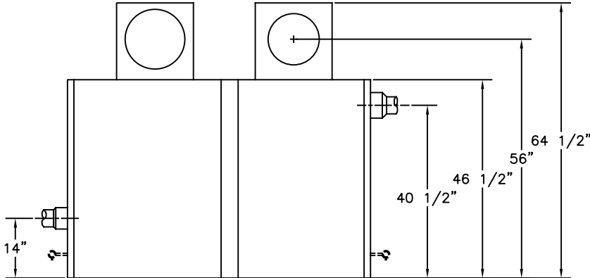
TOP
