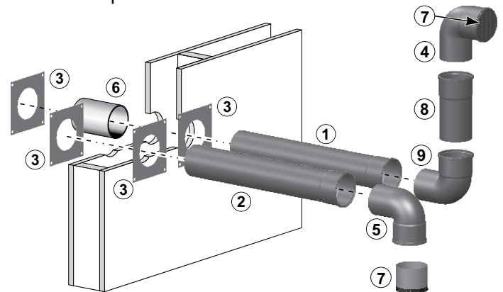
Figure 39 Ensemble de terminaisons dans un mur latéral pour installations à événement direct
