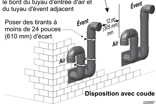
Figure 39 Ensemble de terminaisons dans un mur latéral pour installations à événement direct
