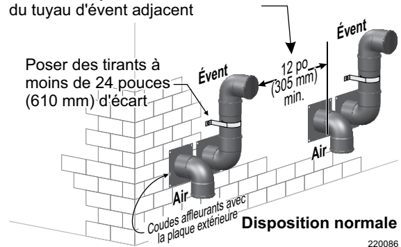
Figure 38 Terminaisons multiples — dégagement entre l'évent d'une terminaison et l'entrée d'air de la suivante
