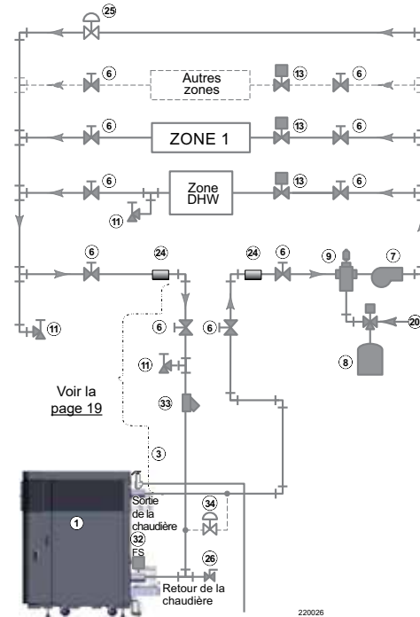
Figure 15 Débit primaire variable avec tuyauterie DHW optionnelle.
