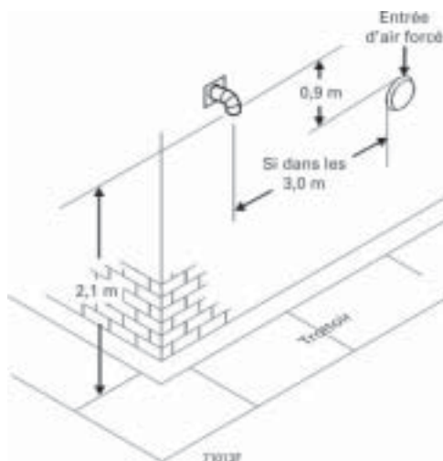
Illustration 12 Dégagements minimum de terminaison d'évent
