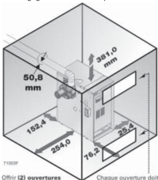
Illustration 2 Dégagements minimum pour les endroits serrés
