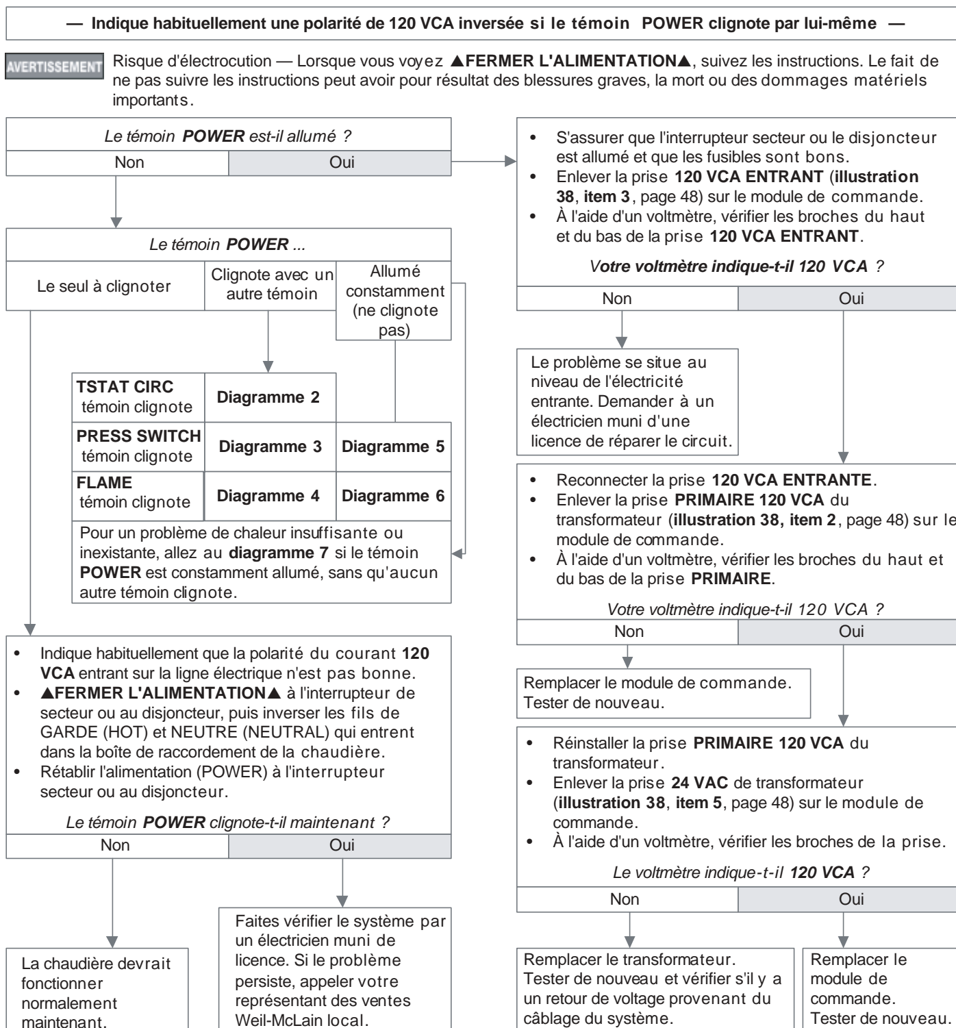
Diagramme 1 — Dépannage de l'état du témoin POWER
