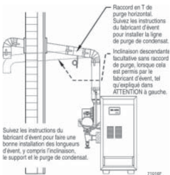
Illustration 14 Évacuation directe évacuation par mur latéral
