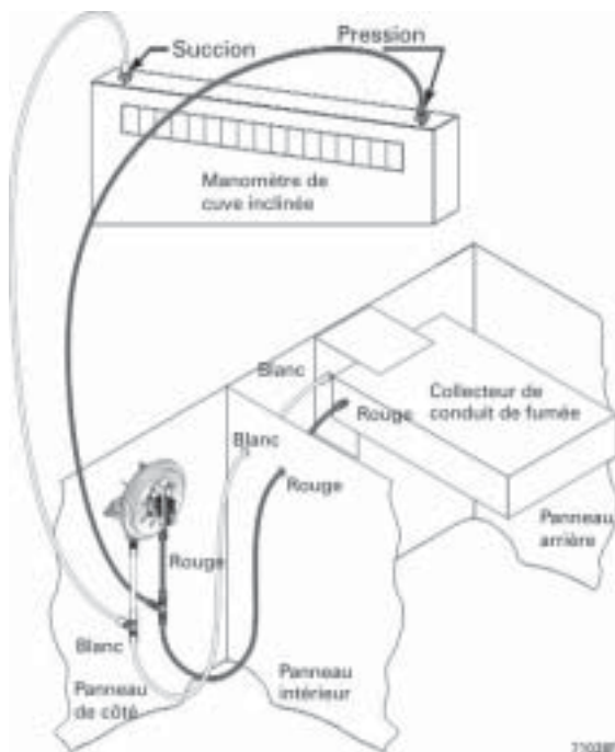
Illustration 36 Connexions de manomètre
