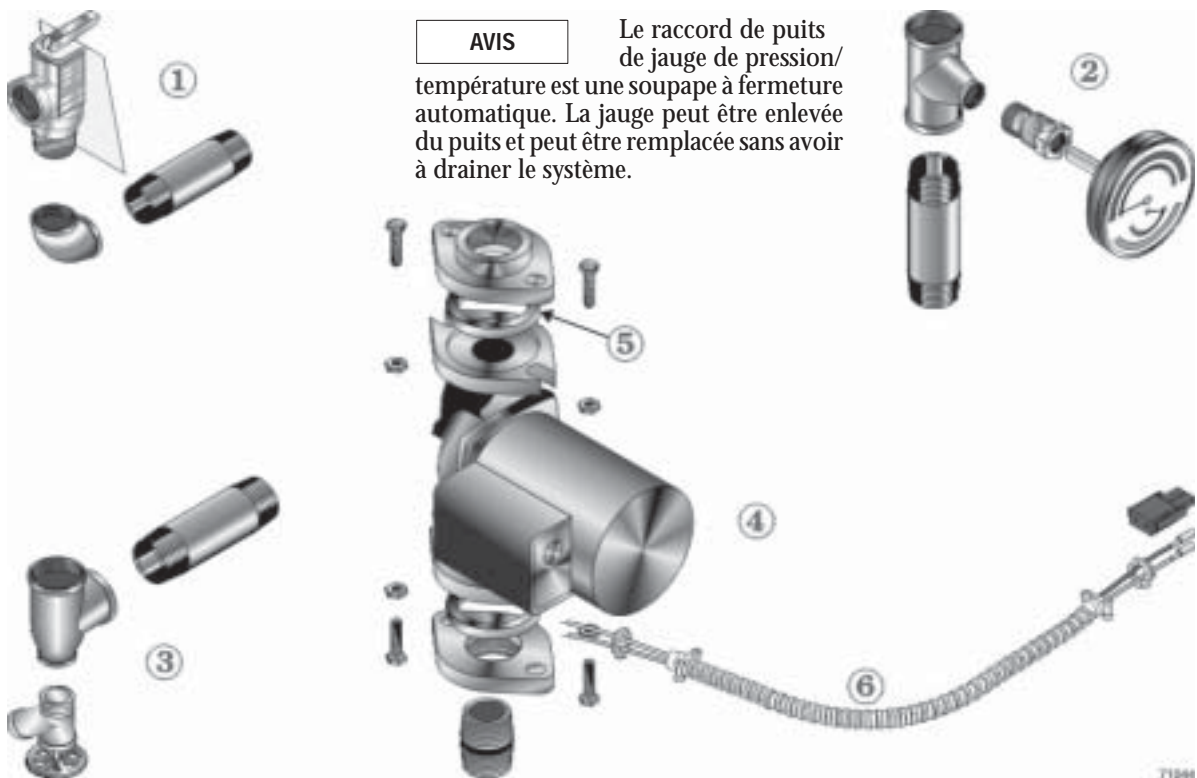
Illustration 42 Pièces d'éléments internes
