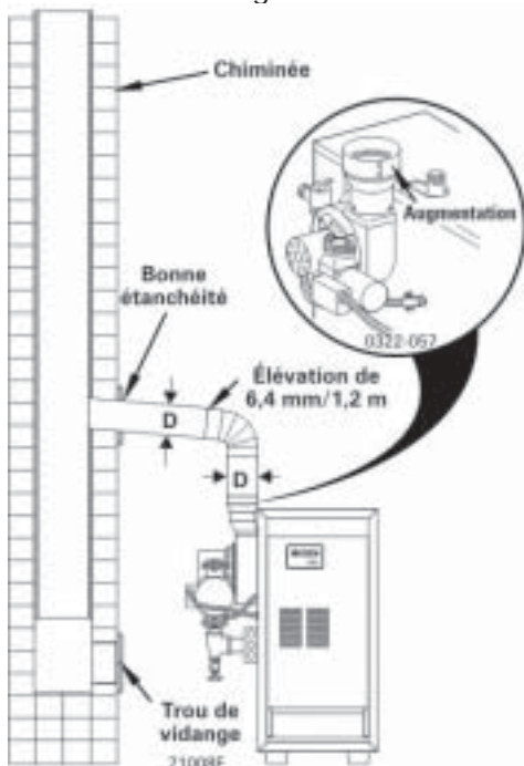
Illustration 7 Évacuation de tirage de cheminée
