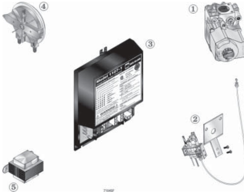
Illustration 43 Pièces de contrôle du gaz
