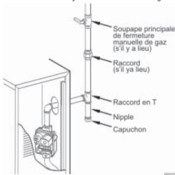
Illustration 26 Tuyauterie d'alimentation en gaz
