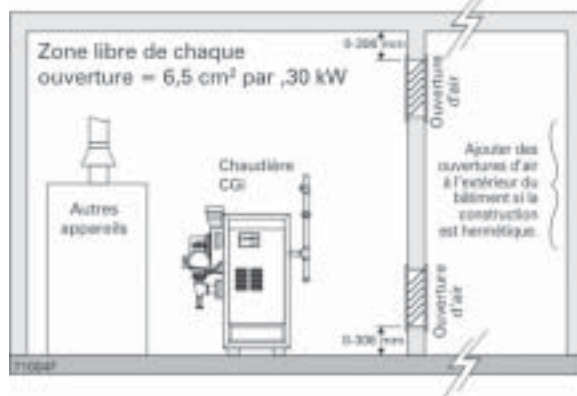
Illustration 3 Ouvertures d'air vers l'espace intérieur
