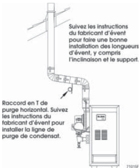
Illustration 13 Évacuation directe évacuation verticale
