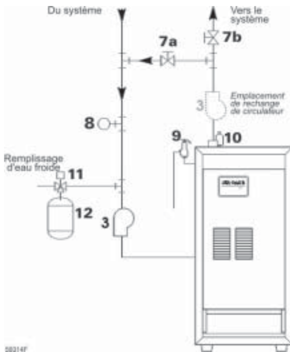
Illustration 24 Tuyauterie de dérivation de système
