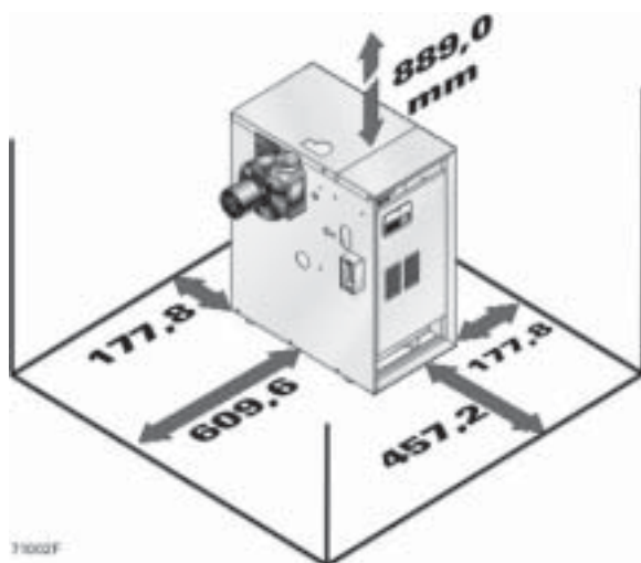
Illustration 1 Dégagements recommandés pour l'entretien
