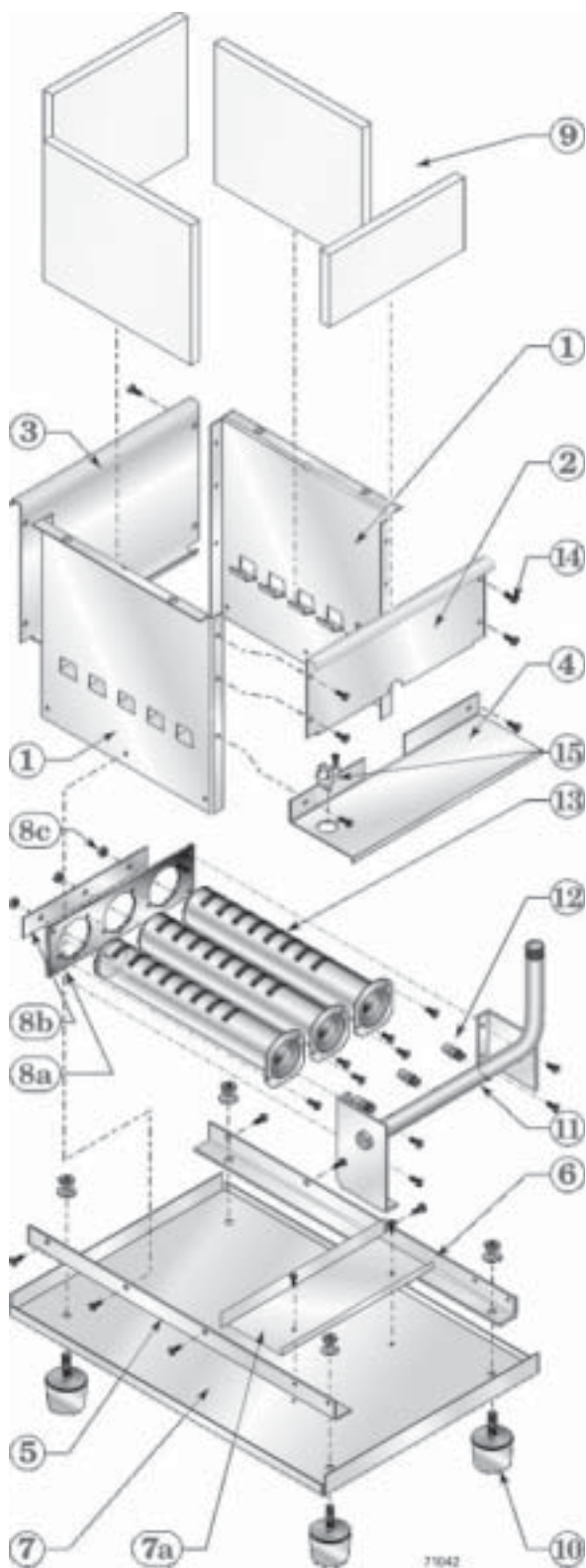
Illustration 40 Pièces de la base
