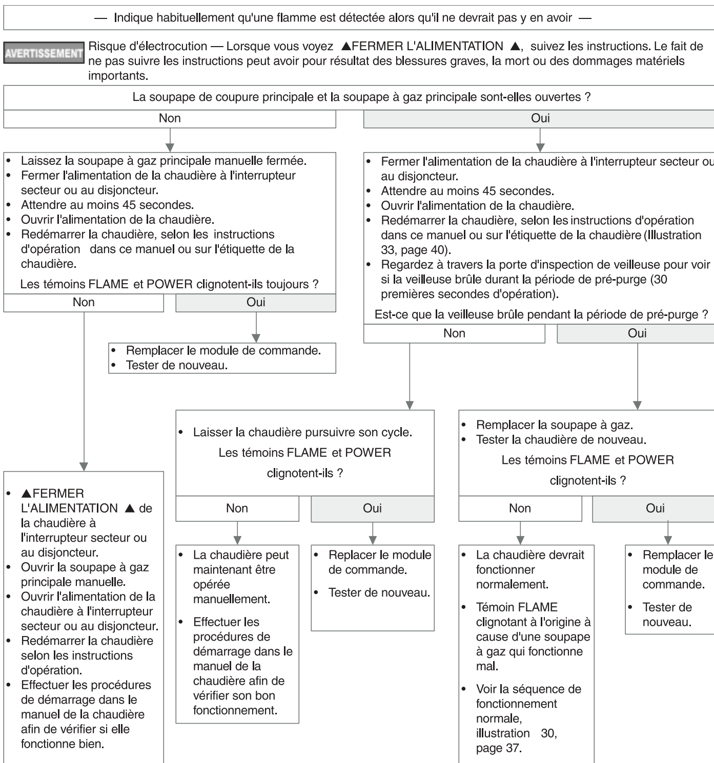
Diagramme 4 — Témoins FLAME et POWER qui clignotent
