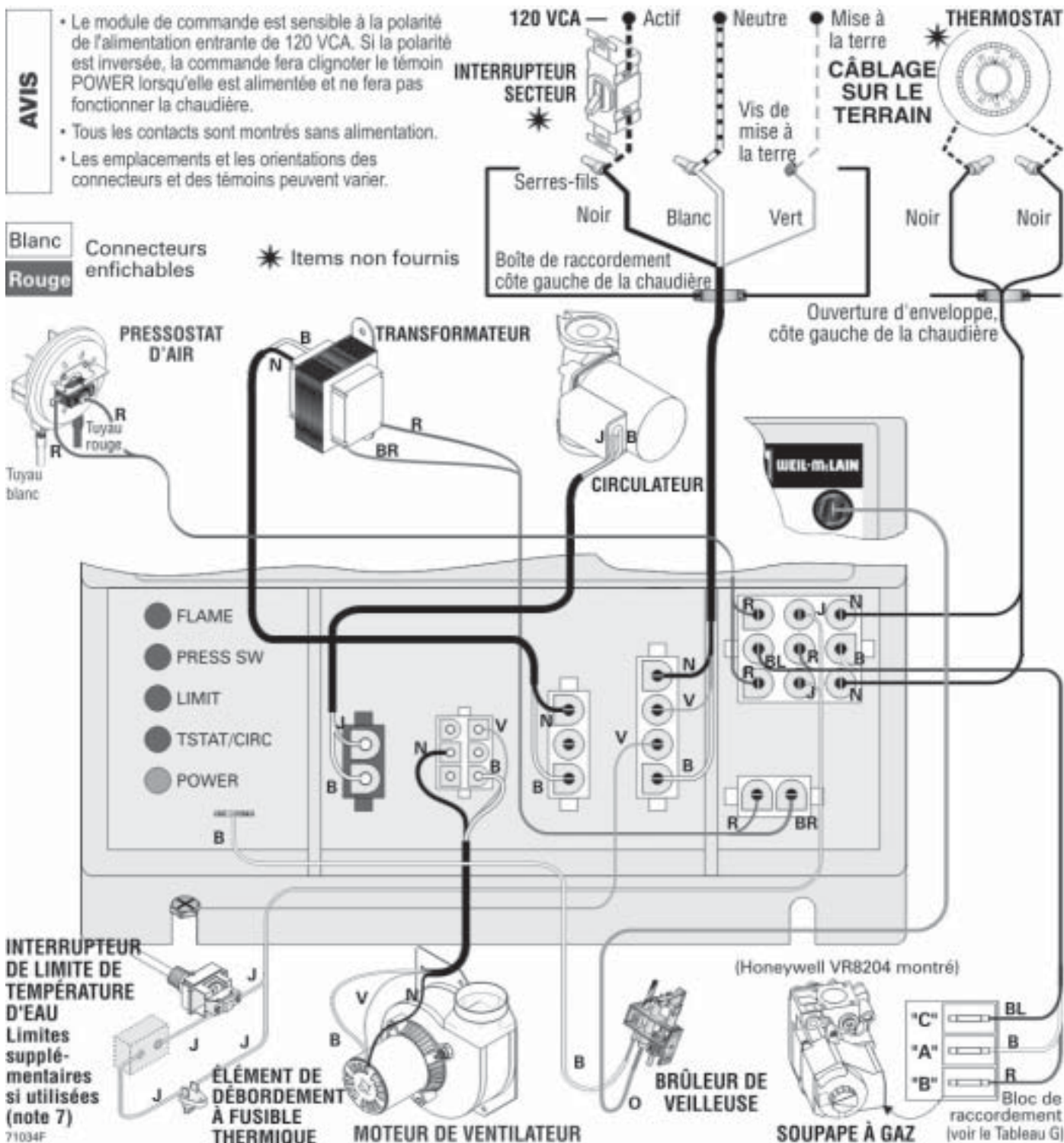
Illustration 31 Schéma de câblage
