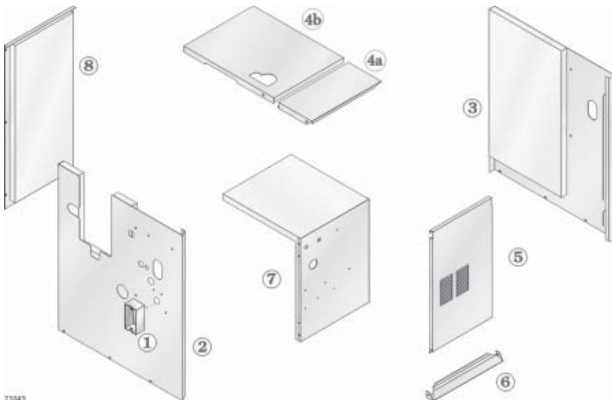
Illustration 41 Pièces de l'enveloppe
