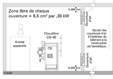
Illustration 3 Air qui provient directement de l'extérieur
