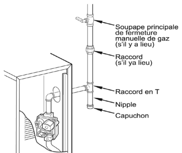
Illustration 26 Tuyauterie d'alimentation en gaz
