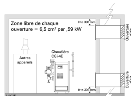
Illustration 5 Air qui provient de l'extérieur — conduits
