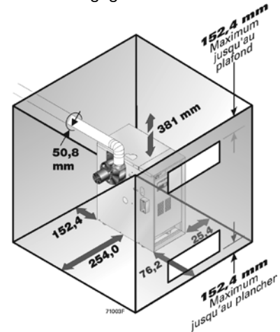
Illustration 1b Dégagements MINIMUM exigés
