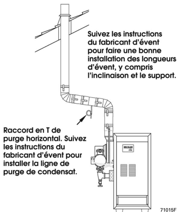
Illustration 13 Évacuation directe évacuation verticale
